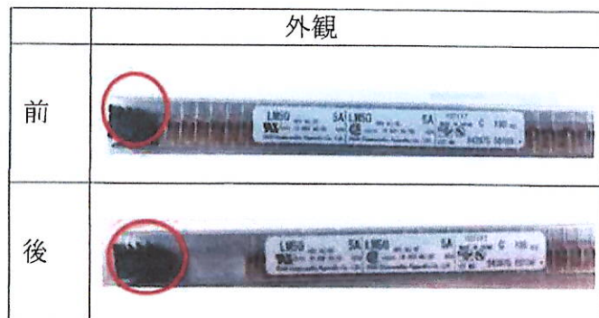
写真2 マイクロヒューズ、ホルダ
