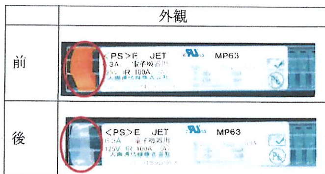
写真1 MP、SDP、MPHストッパー
